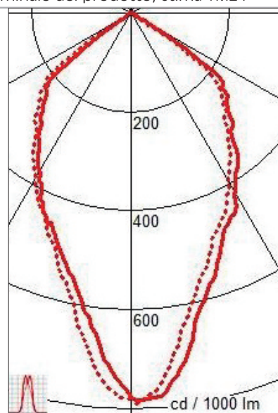
Riflettore 120°
