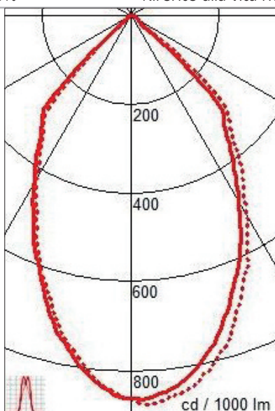
Riflettore 100°
