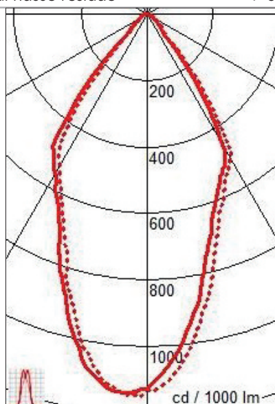
Riflettore 80°
